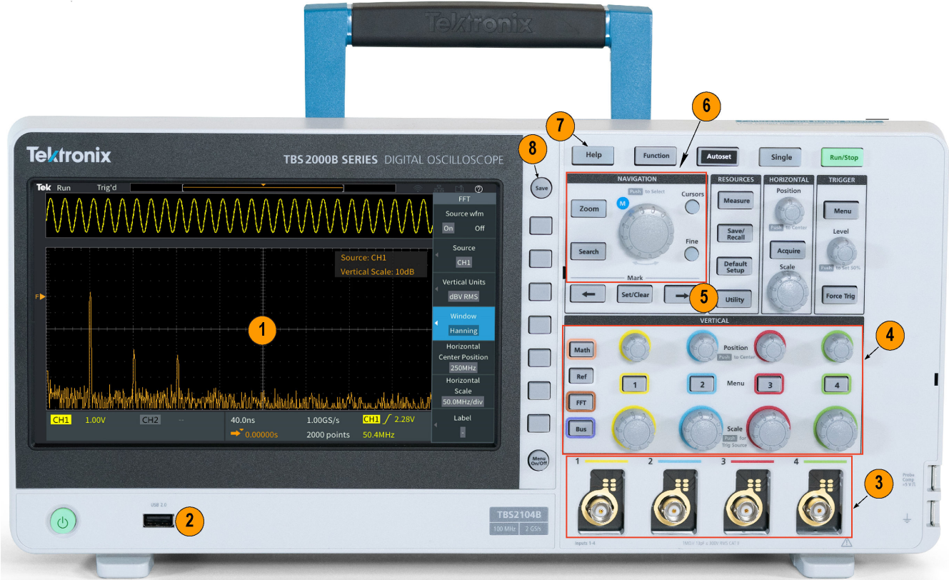
Передняя панель осциллографа TBS2000B
